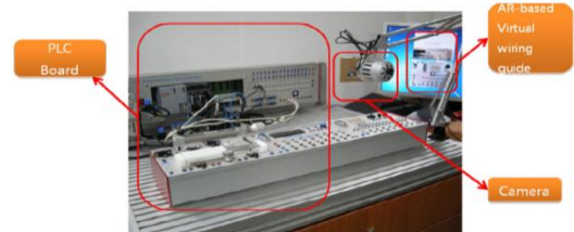
รูปที่ 5 ระบบการเรียนรู้แบบผสมผสาน สำหรับการฝึกอบรมการเดินสายไฟ PLC โดยใช้เทคโนโลยีความจริงเพิ่มเติม (ที่มา: Yoon Sang Kim et al., 2011)
