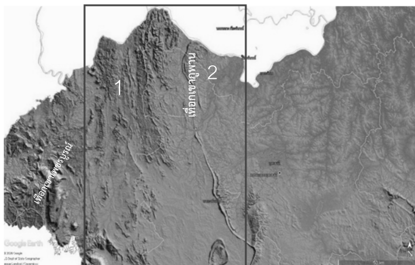
ภาพที่ 2 ภาพถ่ายทางอากาศแสดงลักษณะภูมิประเทศของพื้นที่ ระหว่างลุ่มแม่น้ำเลยถึงห้วยน้ำโมง หมายเลข 1 คือ พื้นที่ฝั่งตะวันตกของเทือกเขาภูพาน หมายเลข 2 คือ พื้นที่ฝั่งตะวันออกของเทือกเขาภูพาน
